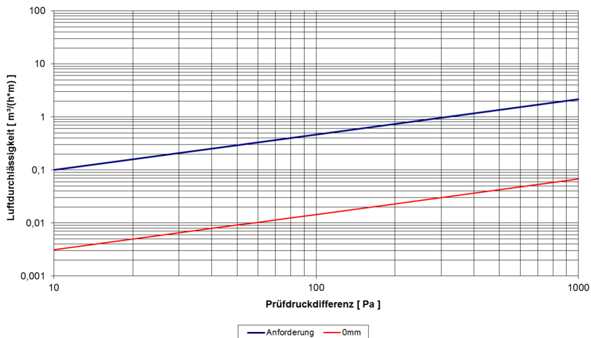
Abbildung 4: Luftdurchlässigkeit (M100)
