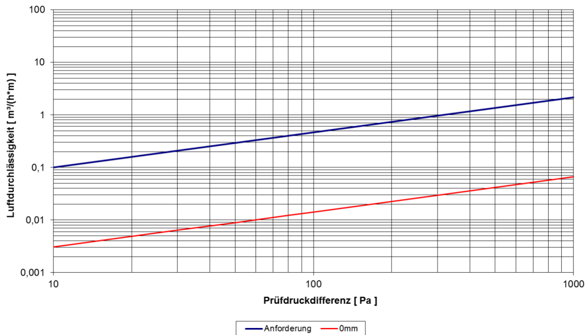
Abbildung 4: Luftdurchlässigkeit (D142)
