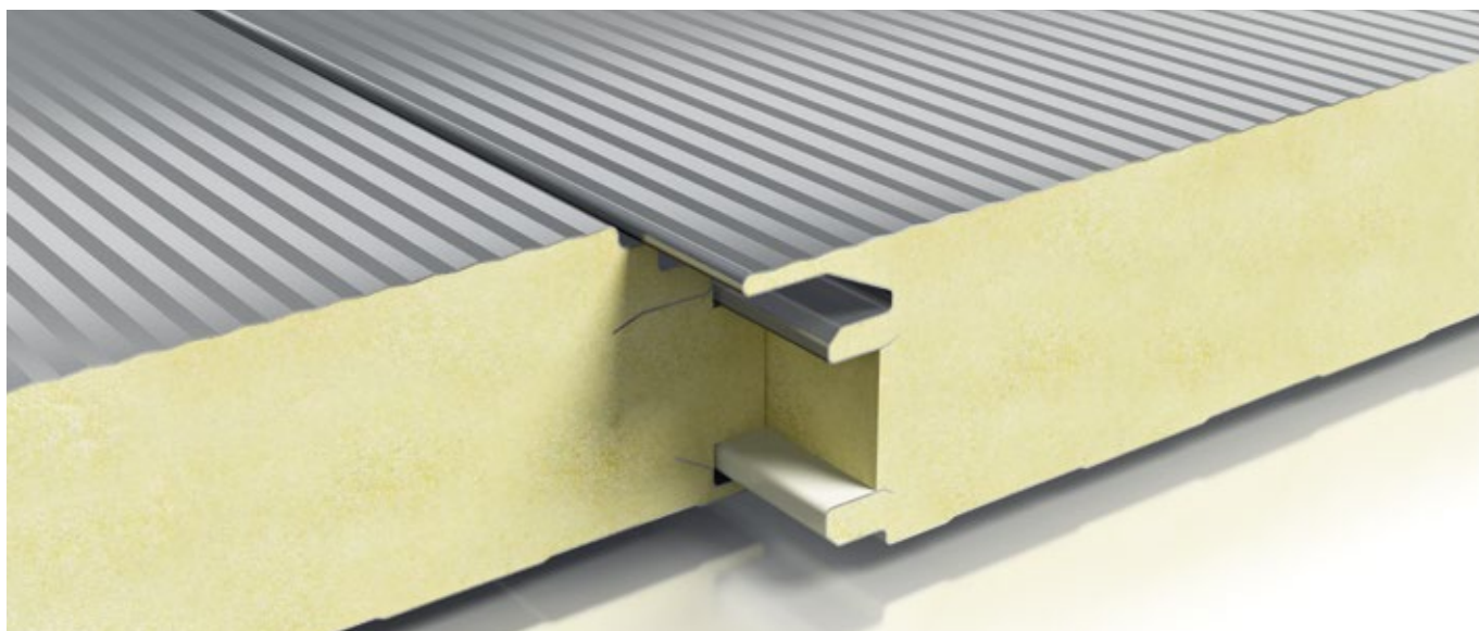
Doppel-Nut-Feder-Verbindung
