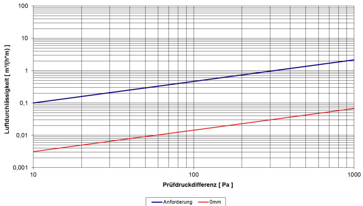
Abbildung 4: Luftdurchlässigkeit (M100)
